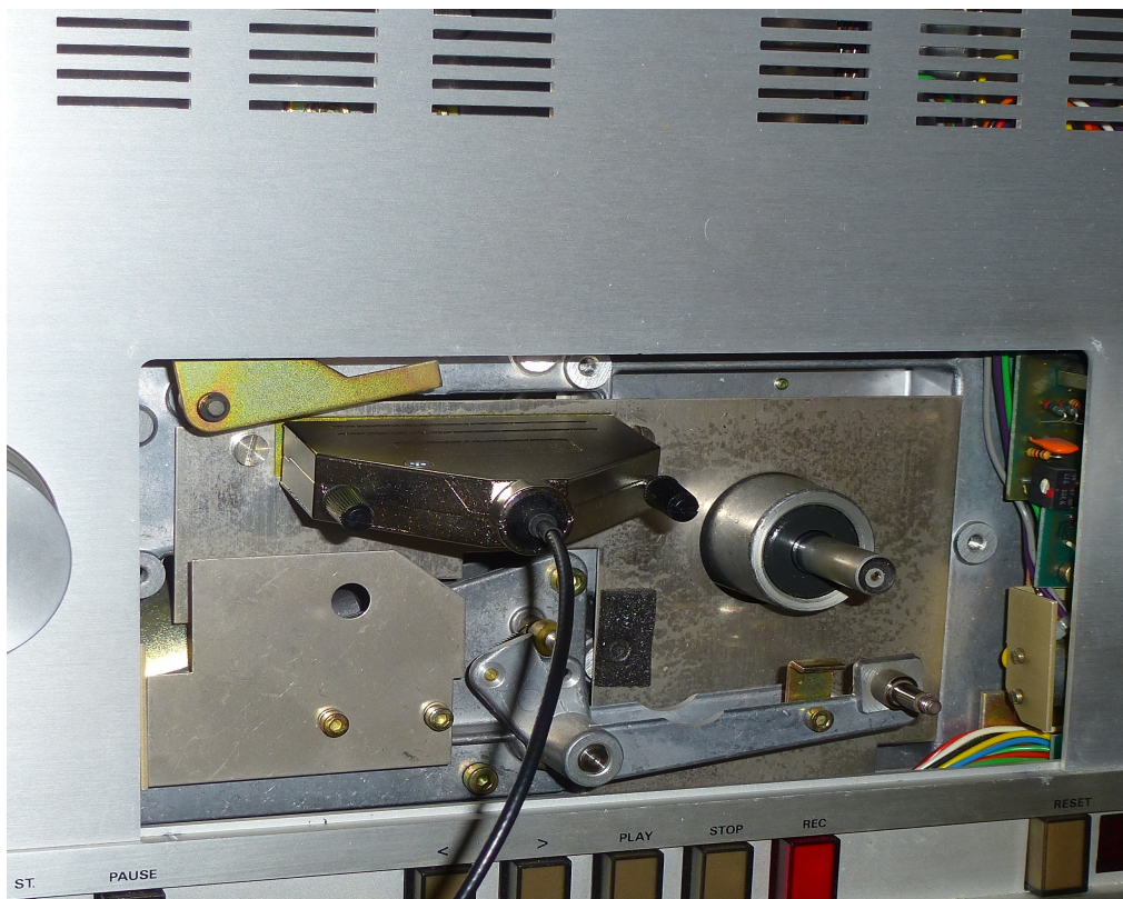
B67 mit Omega-Einspeise-Stecker am Kopfräger -Stecker
